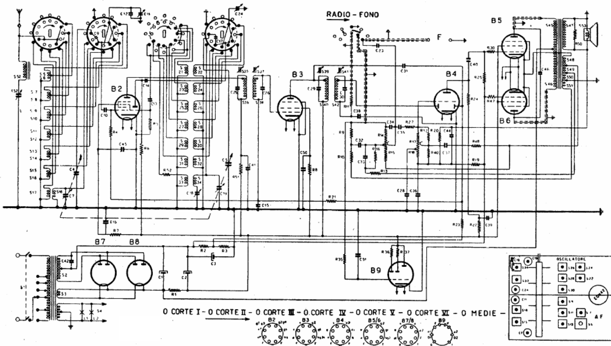
PHILIPS RADIO - Mod. BI 693 A - Onde medie e sei gamme onde corte. Media frequenza 468 kc. Tensione a C1 270 V, a C2 240 V. Corrente anodica totale 73 mA.
