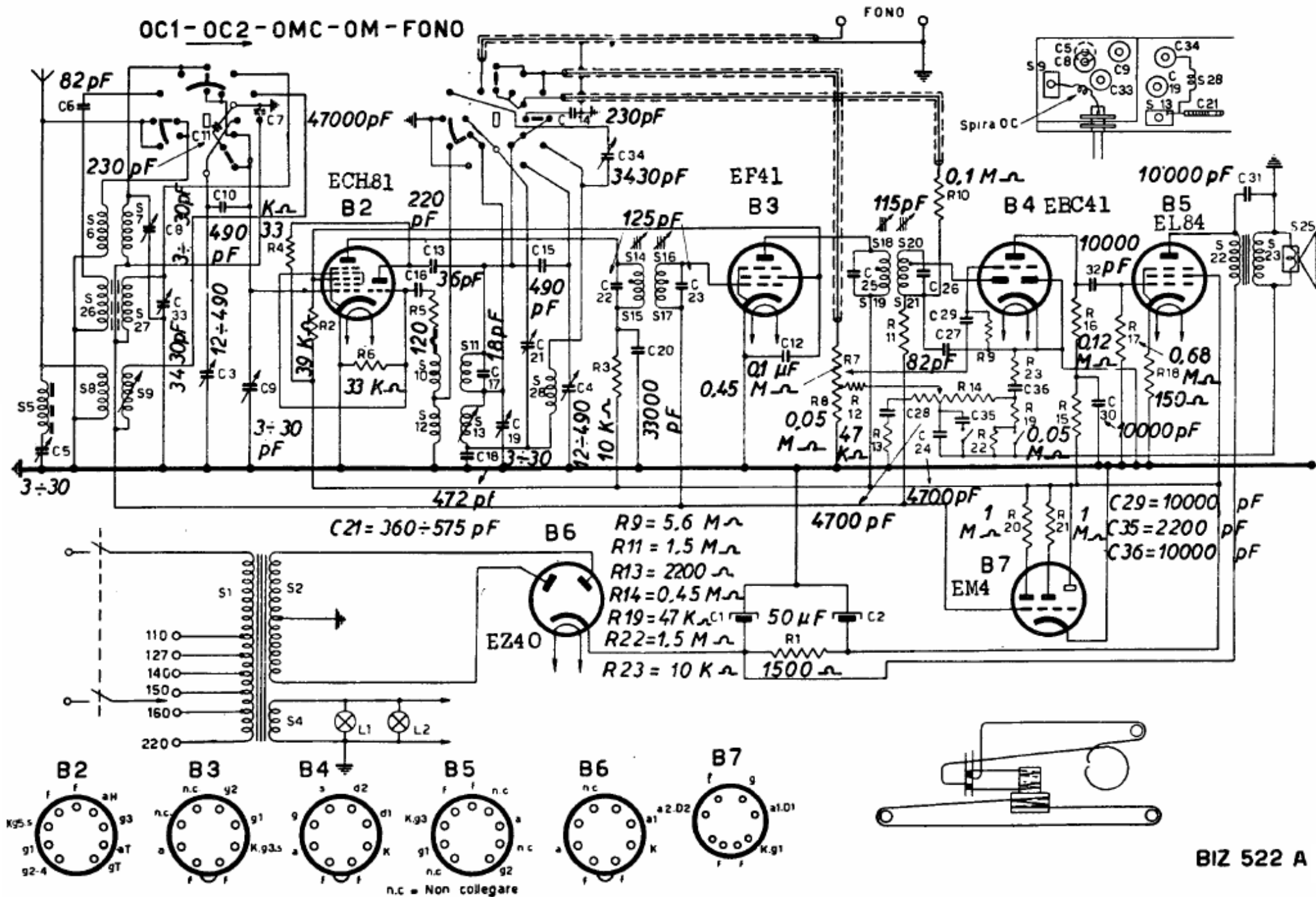
PHILIPS RADIO - Mod. BIZ 522 A. Quattro gamme d'onda: onde medie da 1630 a 517 kc/s; onde medio-corte da 3,1 a 1,6 Mc/se due gamme onde corte, compresa quella per pescherecci. Media frequenza 468 kc/s. Corrente anodica totale 60 mA. Consumo 44 watt.
