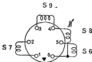
Oscillateur FK 850 24
