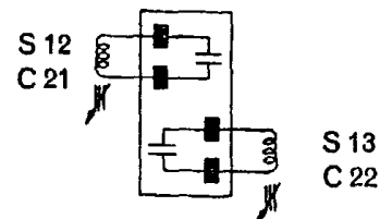
Transfo MF 2 FD 003 26
