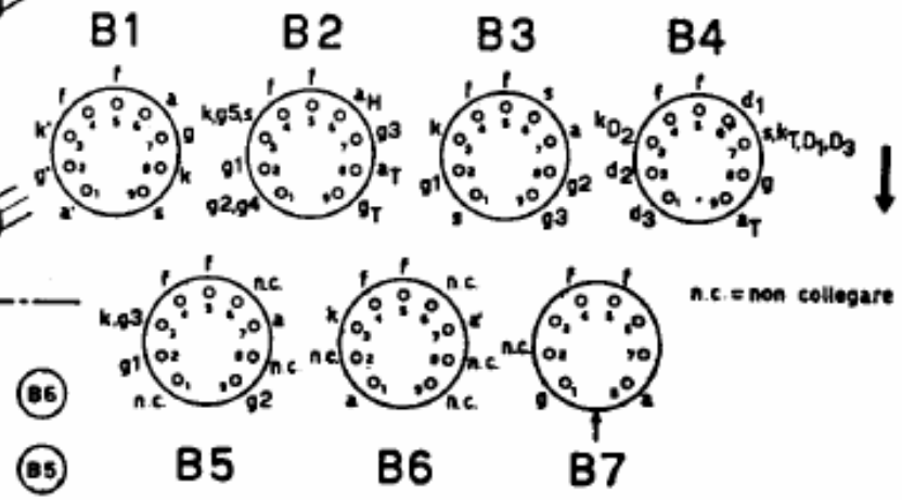
PHILIPS RADIO - Mod. BI 361 Alfieri. Apparecchio a modulazione d'ampiezza e di frequenza, con una gamma onde medie, una gamma onde corte e una gamma onde ultracorte. Media frequenza AM a 460 kc/s. Media frequenza FM a 10,7 Mc/s.
