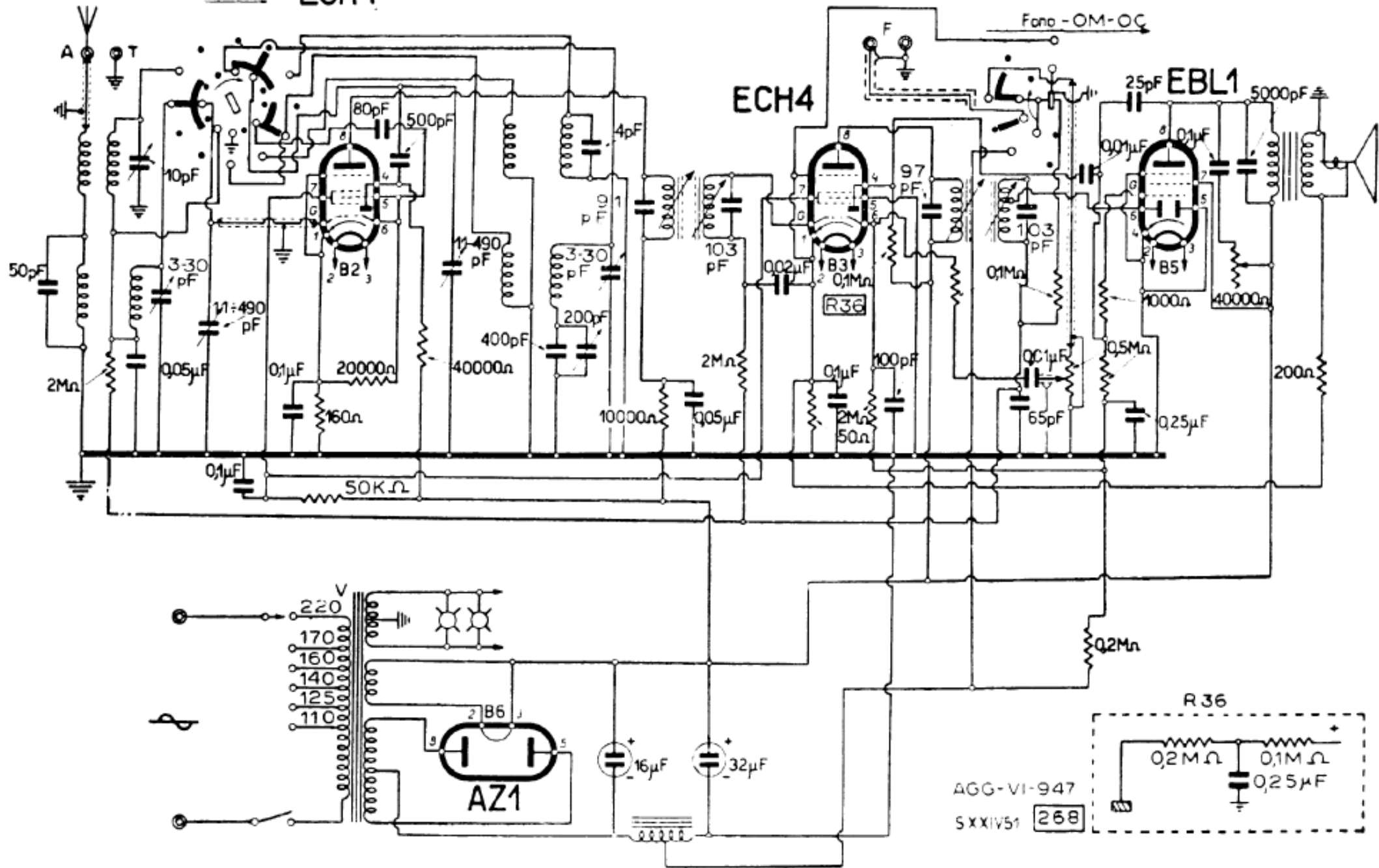
Lo schema elettrico dei modd. BI 460 A - B! 471 A - HI 470 A.
