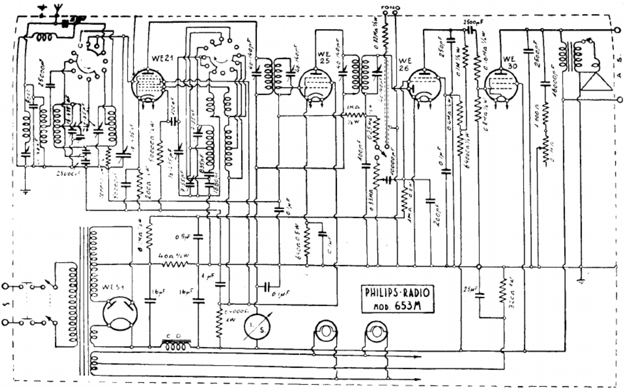
129. — PHILIPS RADIO. — Modello « 653 M ». — Produzione 1937-1938. — Media frequenza: 115 kHz.
