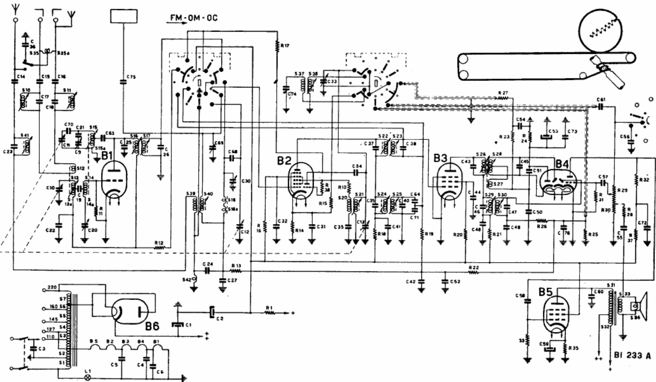
PHILIPS RADIO - Mod. BI. 233 A. Apparecchio a modulazione di ampiezza e di frequenza. Una gamma onde medie AM (da 517 a 1630 kc/s), una gamma onde corte AM (da 5,9 a 11,5 Mc/s) ed una gamma onde ultracorte FM (da 80 a 108 Mc/s). Media frequenza AM 460 kc/s; media frequenza FM 10,7 Mc/s.
