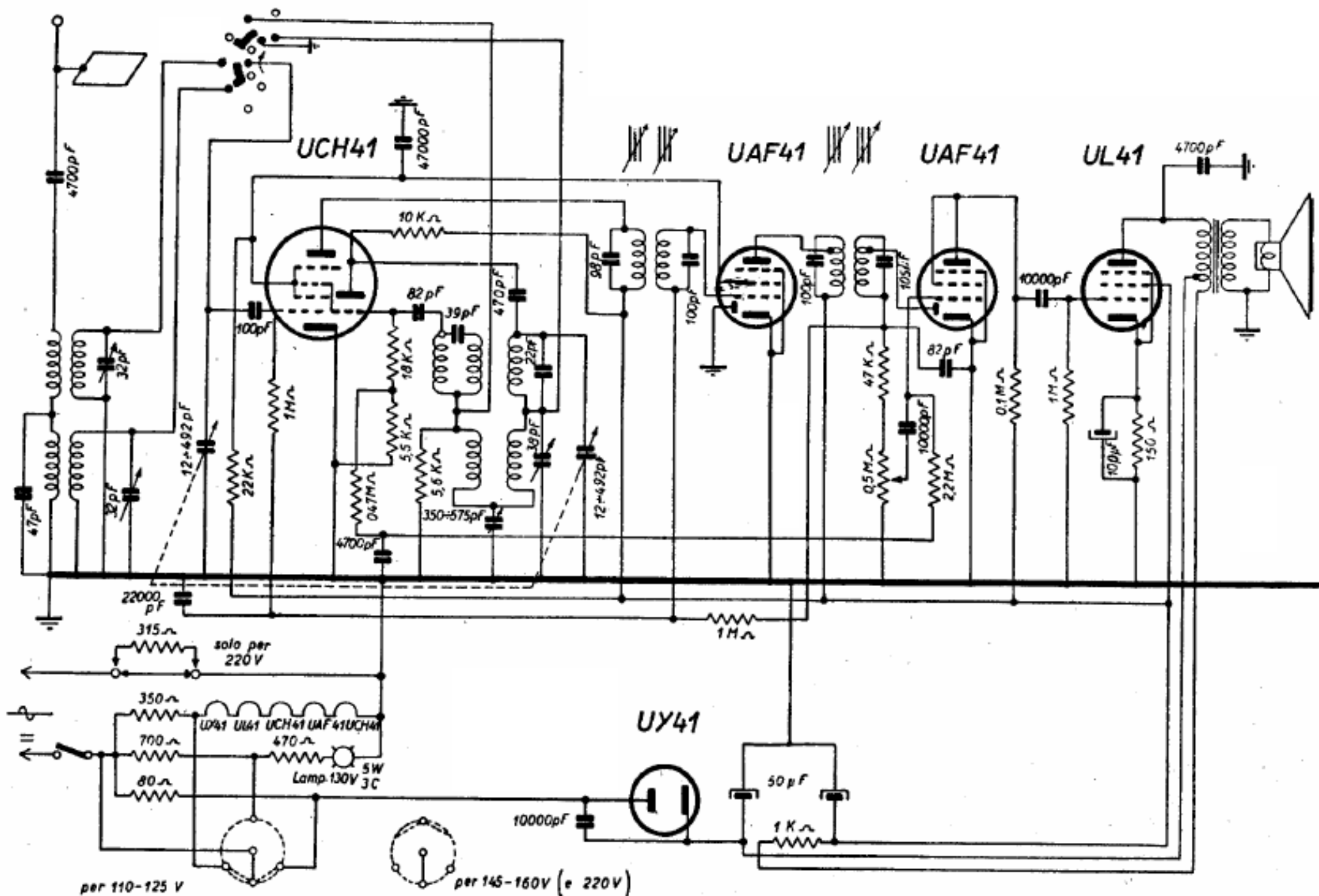
PHILIPS RADIO - Modd. BI 281 U e BI 290 U - Medie e corte. Media frequenza a 468 kc. Placca finale 135 V e 44 mA, schermo 131 V e 6,5 mA. Altre placche 130 V, schermi 75 V. Corrente anodica totale 64 mA.
