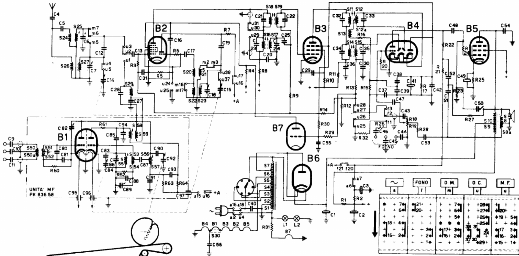
COMMUTATORE IN POSIZIONE O.C.
