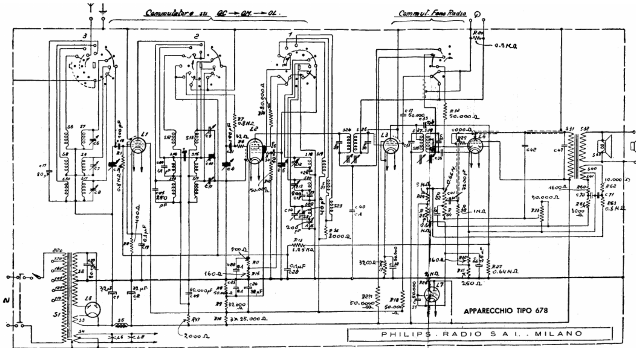
[ PHILIPS RADIO - Mod. « 678 e 682 » - Produzione 1939-1940. - Valvole: L1 = EF8, L2 = EK2, L3 = EF9, L4 = 6BL1, L5 = W154, L7 = EM1. - Gamma: c. c. (16,5-32 m), c. (28-50 m), m. (180-580 m), l. (700-2000 m). Media frequenza: 488 kHz. - Sintonizzazione automatica per 8 stazioni. - Potenza: 2 watt. (V. anche per la parte alta e media frequenza il mod. 744). - (C42 = 5000 pF, C47 = 2000 pF).
