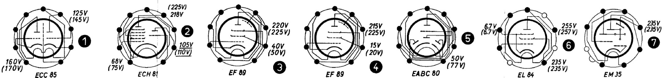
gezeichnete Schalterstellung: UKW Taste gedrückt.
