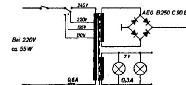
Entgegen dem Trafoschema ist 150 V Netzanschluß vorhanden.
