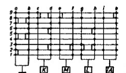
gezeichnete Schalterstellung: UKW Taste gedrückt.
