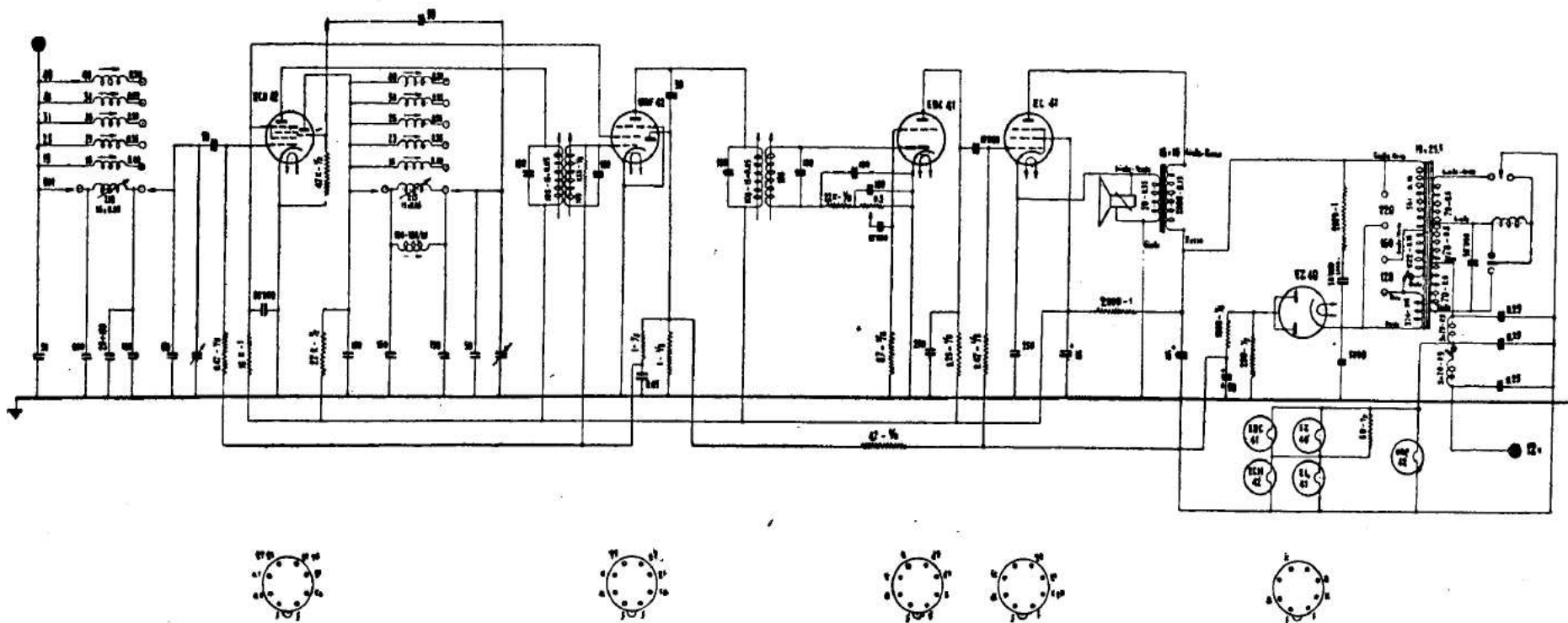
ASTER RADIO - Mod. 506 - Apparecchio radio da automobile. Media frequenza 468 kc. Onde medie e bande allargate a 19, 25, 31, 41 e 49 metri. Resa d'uscita 3 watt.
