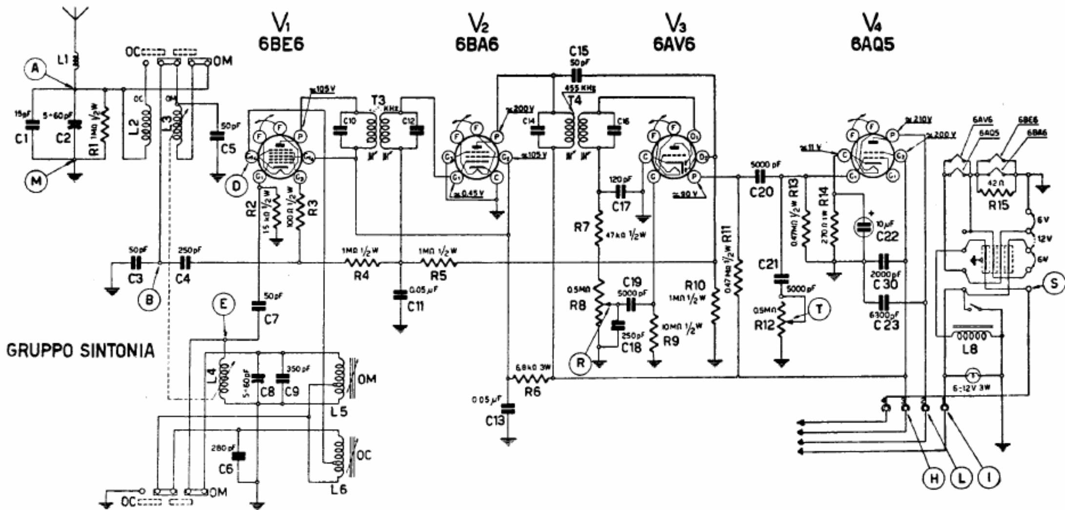
AUTOVOX - Mod. RA 49 prima serie. Onde medie da 520 a 1600 kc/s e onde corte da 5,95 a 6,3 Mc/s. Media frequenza a 455 kc/s. Potenza d'uscita circa 1 watt. Consumo totale: 2,3 A a 13,5 V e 4,6 A a 6,75 V. (V. schema alimentatore a parte).
