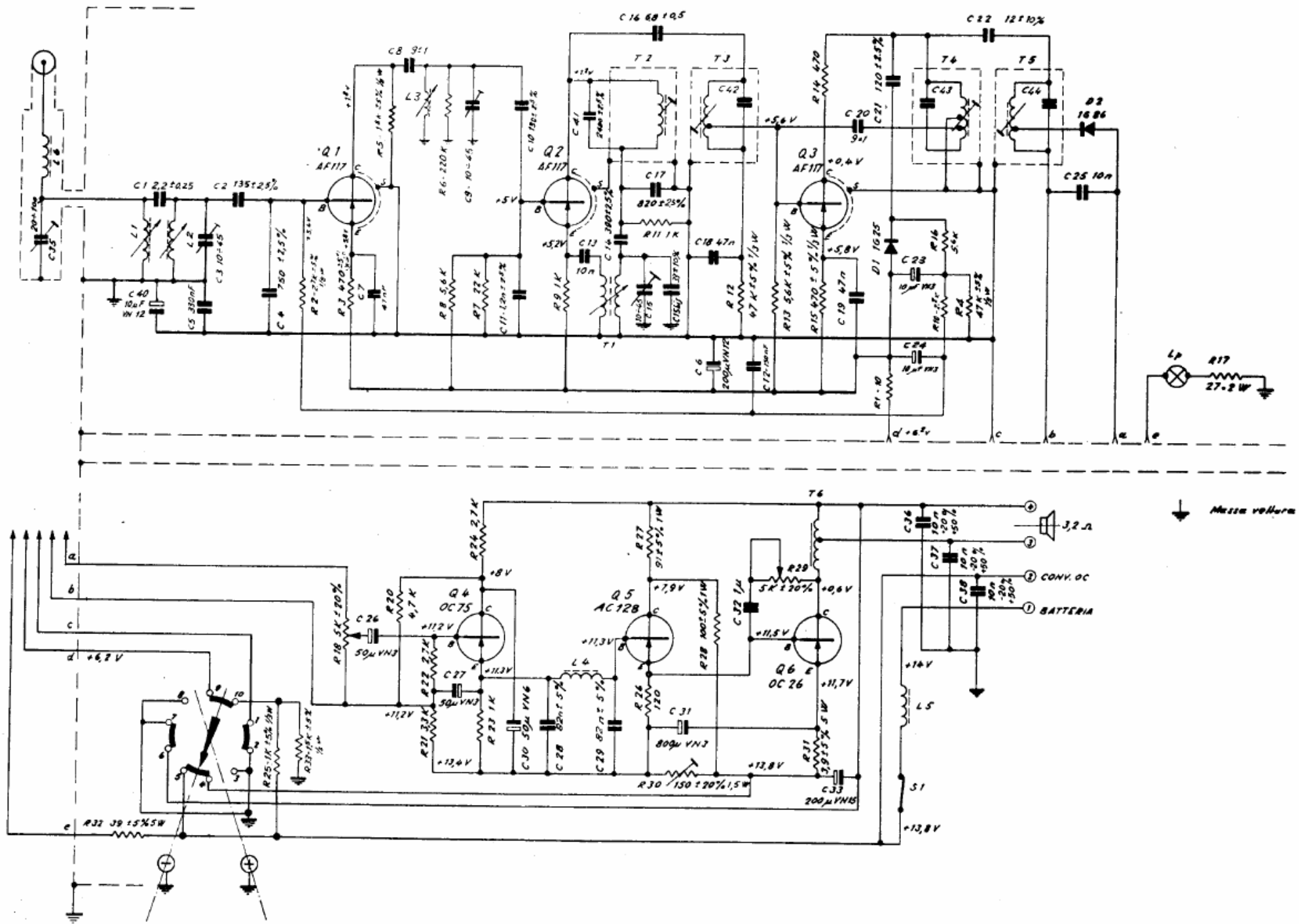
AUTORADIO AUTOVOX Modd. RA 441 - 442 - 443 - 444 - 445 - 446 .
